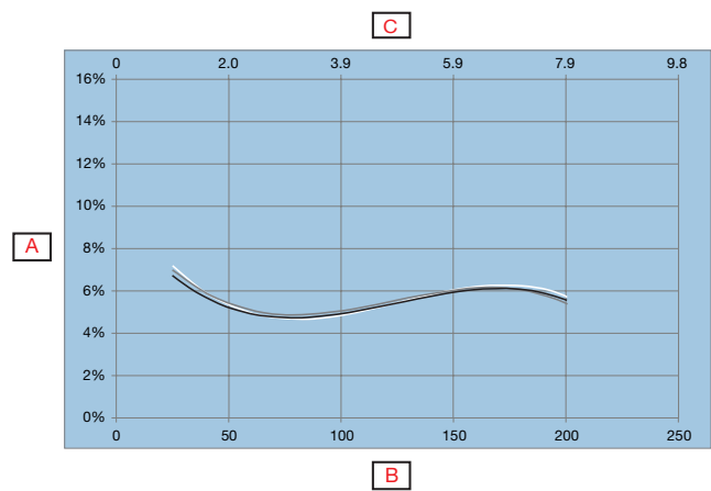
Fig. 5 PD30ETBI20BPxxIO
